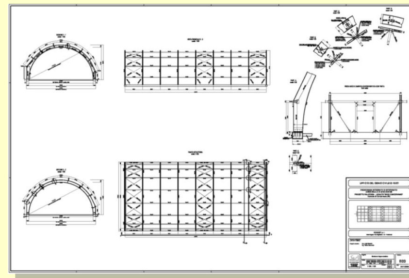
Sezioni, prospetti e planimetria Impianto sportivo Polivalente
